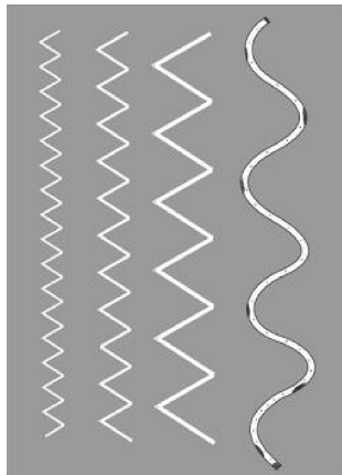
Gambar 2 Motif Lajur
