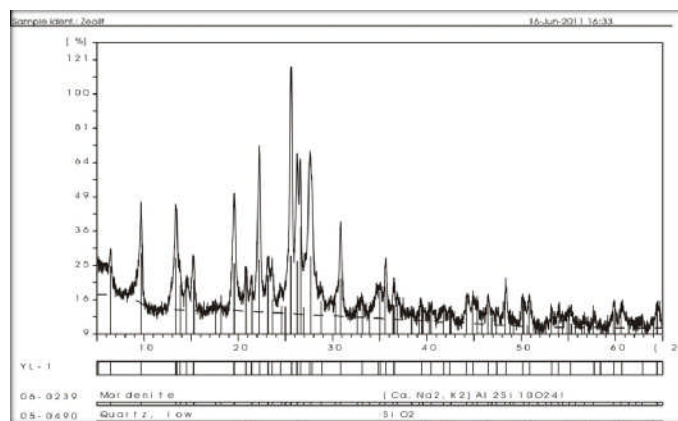
Gambar 1. Hasil Uji XRD Sampel Zeolit
