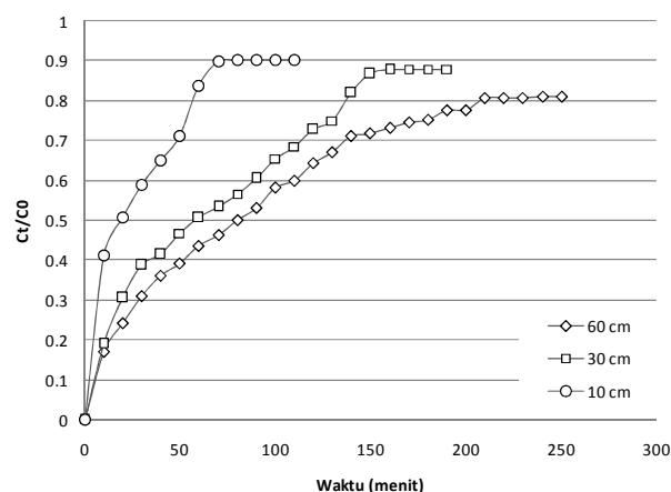
Gambar 4. Kurva Breakthrough Pengaruh Tebal Adsorben Terhadap Efektifitas Penyisihan Warna pada Limbah Cair Sasirangan
