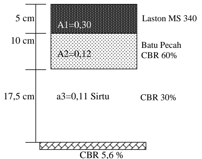
Gambar 3. Tebal Perkerasan metode NCSA
