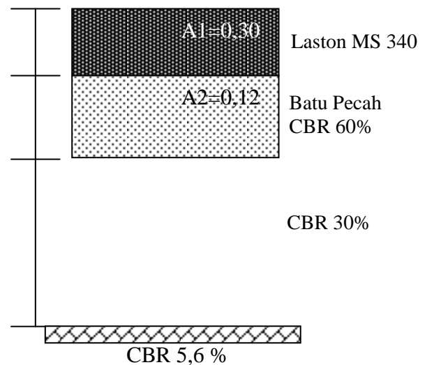
Gambar 1. Tebal Perkerasan Metode Analisa Komponen Bina Marga
