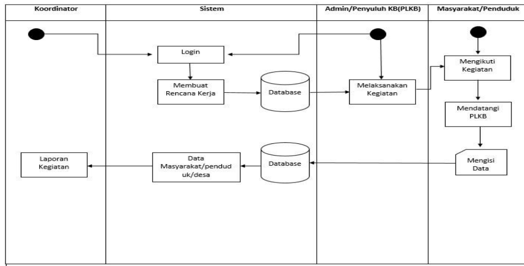
Gambar 2. Flowchart sistem yang dibuat
