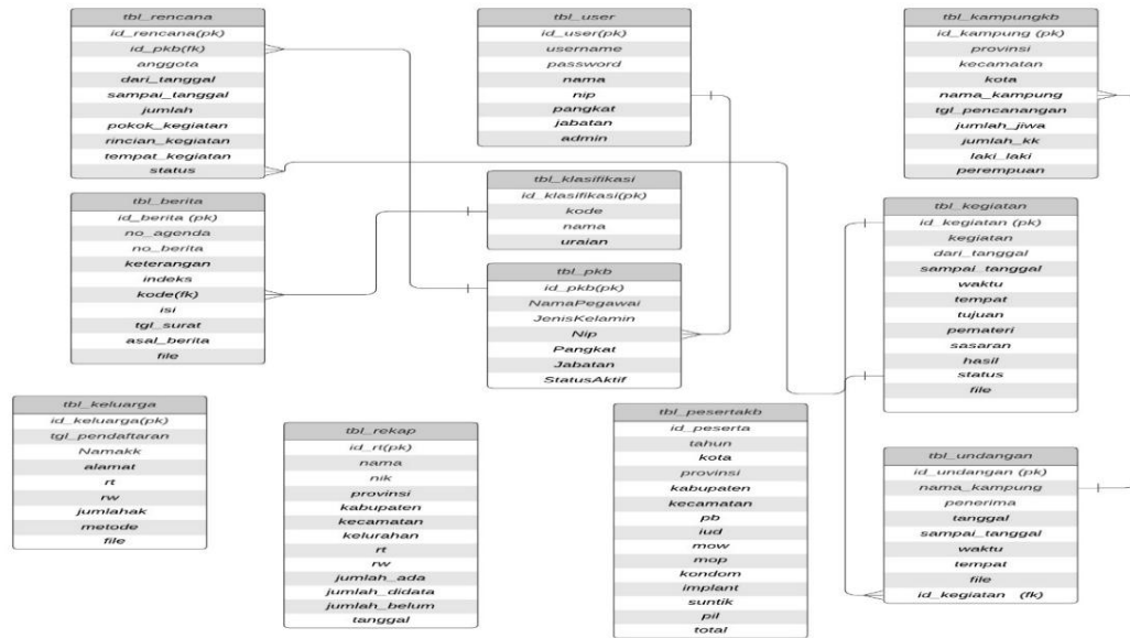
Gambar 3. Desain Relasi Tabel
