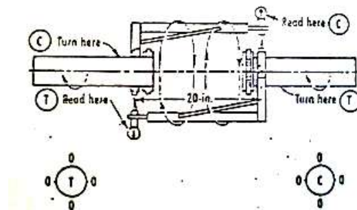
Gambar 1. Bentuk shaft dalam keadaan lurus sempurna
