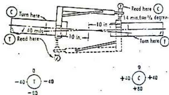
Gambar 4. Bentuk shaft dalam keadaan kombinasi misalignment
