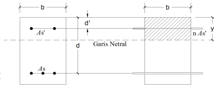
Gambar 2.3 Penampang Transformasi
