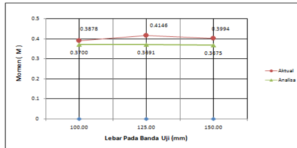
Gambar 3.3 Kurva hubungan rasio b/h dengan momen.
