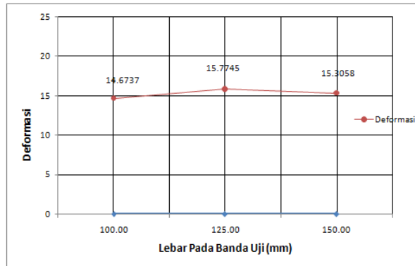
Gambar 3.5 Kurva hubungan rasio b/h dengan deformasi
