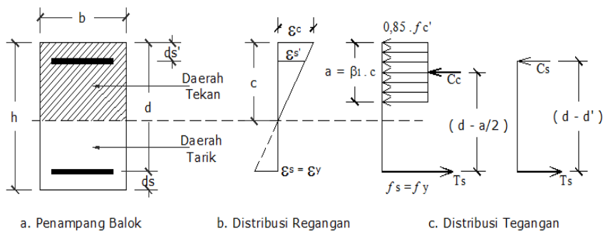
Gambar. 2.1 Distribusi Tegangan Regangan Balok Bertulangan Rangkap.
