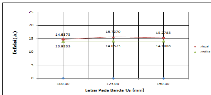
Gambar 3.4 Kurva hubungan rasio b/h dengan Defleksi
