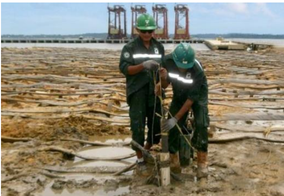
Gambar 53. Pemasangan vibrating wire pm.
