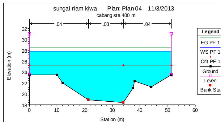
Gambar 3. Hasil Running HEC-RAS untuk Kala Ulang 2 Tahun
