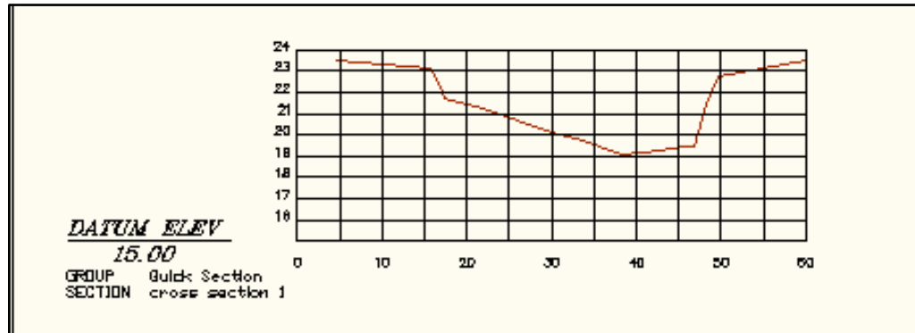
Gambar 2. Hasil Penggambaran Penampang Sungai.
