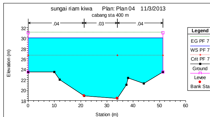
Gambar 4. Hasil Running HEC-RAS untuk Kala Ulang 100 Tahun
