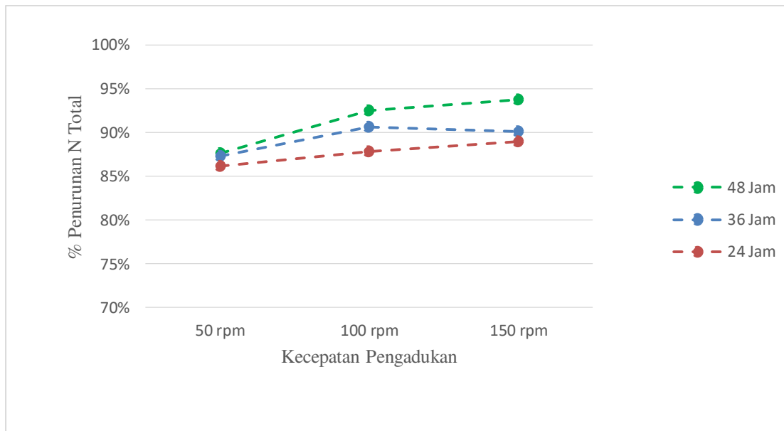
Gambar 7. Hubungan Kecepatan Pengadukan dengan % Penurunan N Total Pada Penambahan Impeller
