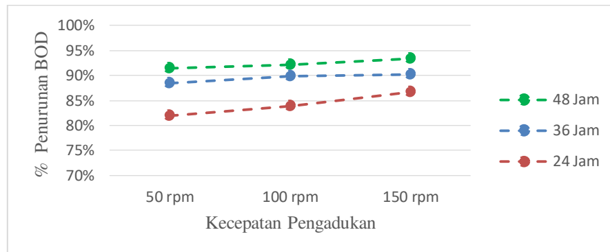
Gambar 5. Hubungan Kecepatan Pengadukan dengan % Penurunan BOD Pada Penambahan Impeller
