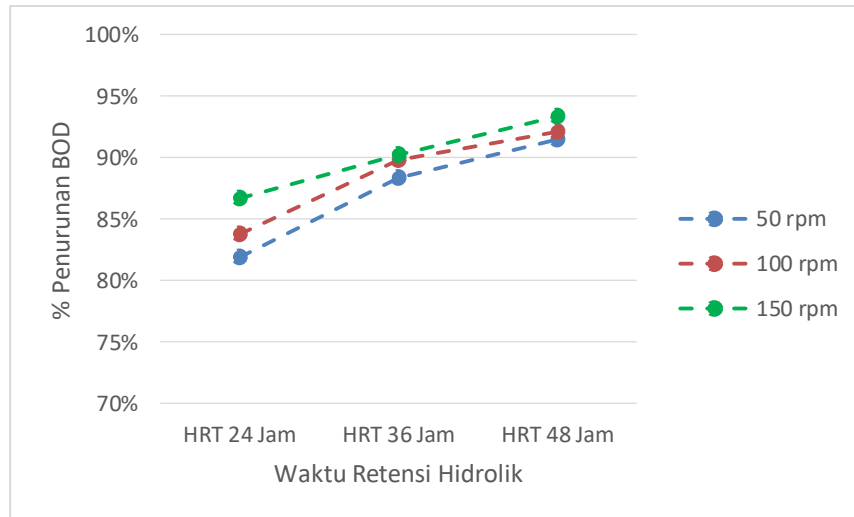
Gambar 2. Hubungan Waktu Retensi Hidrolik terhadap % Penurunan BOD Pada Penambahan Impeller
