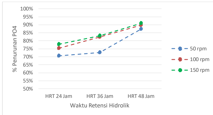
Gambar 3. Hubungan Waktu Retensi Hidrolik terhadap % Penurunan PO 4 Pada Penambahan Impeller
