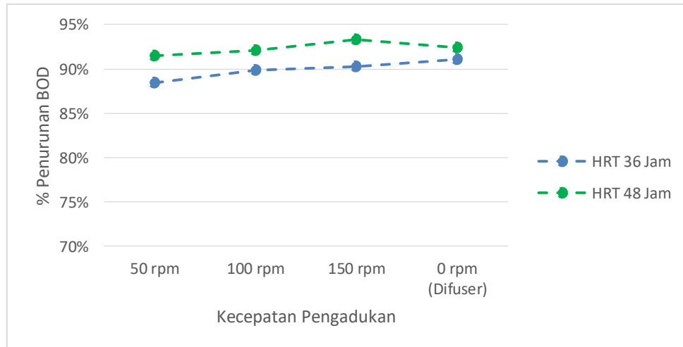
Gambar 8. Grafik Hubungan Kecepatan Pengadukan Terhadap Penurunan BOD
