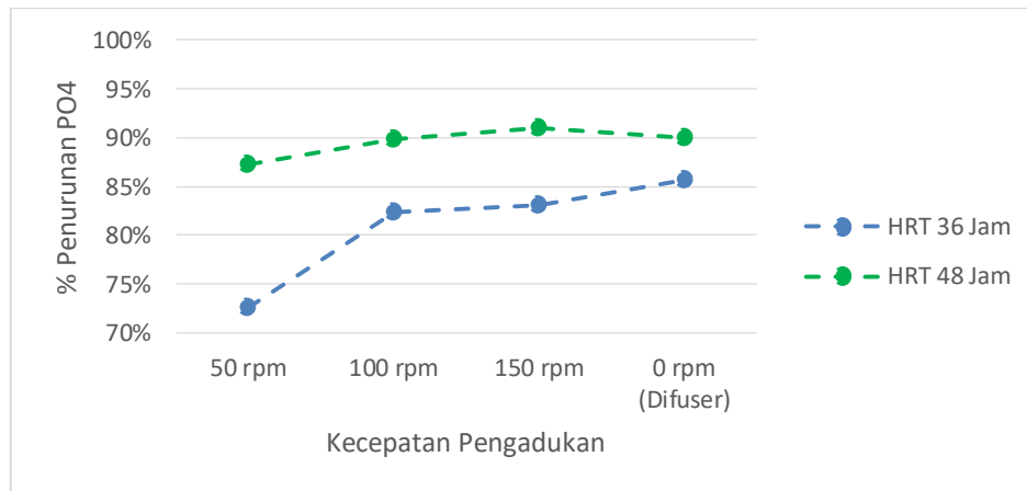
Gambar 9. Grafik Hubungan Kecepatan Pengadukan Terhadap Penurunan PO_4
