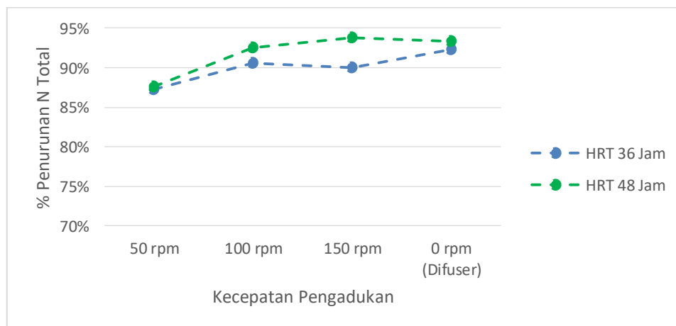
Gambar 10. Grafik Hubungan Kecepatan Pengadukan Terhadap Penurunan N Total
