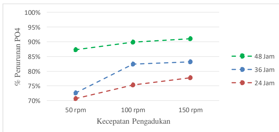
Gambar 6. Hubungan Kecepatan Pengadukan dengan % Penurunan PO_4 Pada Penambahan Impeller
