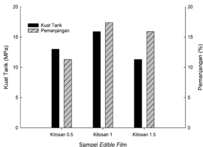
Gambar 3. Analisa Kuat Tarik dan Pemanjangan Pemutusan
