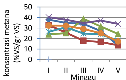
Gambar 3. Pengaruh volatile solid pada pembentukan metana
