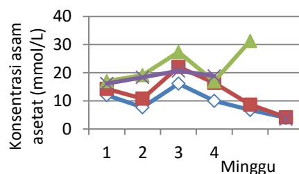
Gambar 4. Konsentrasi asam asetat pada tiap digester dengan %VS yang berbeda pada tiap digester
