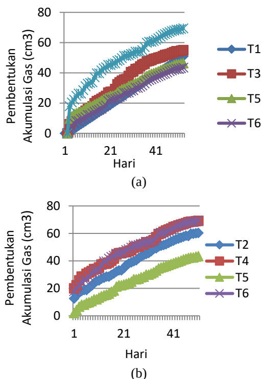
Gambar 2. Pengaruh volatile solid terhadap Pembentukan Akumulasi Volume Biogas, (a). T1 dan T3 yang memiliki %VS sama, yaitu 15%VS akumulasi gasnya tidak sama, (b). T1 dan T3 yang memiliki %VS sama, yaitu 20%VS akumulasi gasnya tidak sama, T4 akumulasi gas lebih besar
