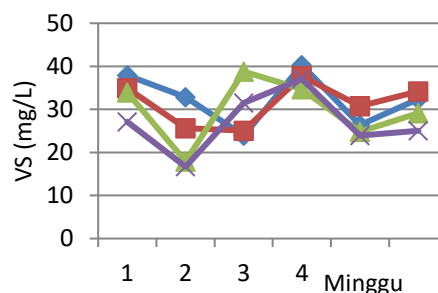
Gambar 5. Pengaruh konsentrasi volatile solid pada produksi volatile fatty acid (VFA) sebagai asam asetat dari beberapa digester
