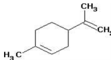
Gambar 1. Rumus bangun limonene
