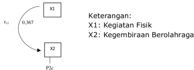
Gambar 2. Model hipotesis pertama setelah dilakukan uji regresi
