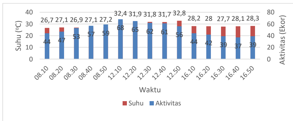
Gambar 1. Hubungan Waktu Pengukuran Suhu Udara Terhadap Jumlah Individu Lebah Kelulut yang Beraktivitas pada Area Stup
