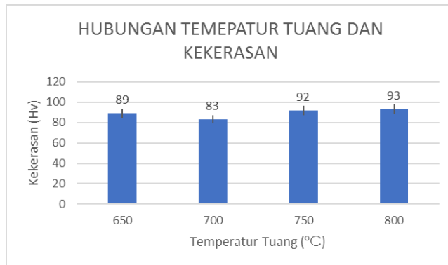
Gambar 17. Hasil Pengujian Kekerasan Baling – baling Surabaya
