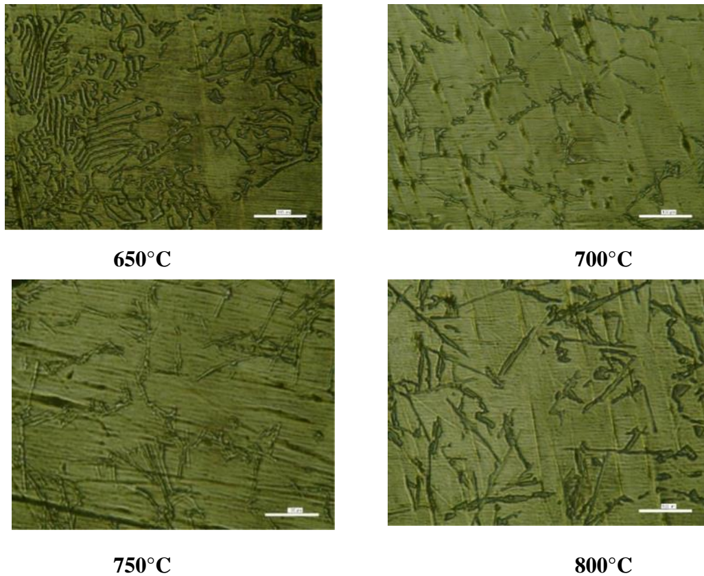
Gambar 15. Hasil Pengujian Struktuk Mikro Baling – Baling Kapal Negara
