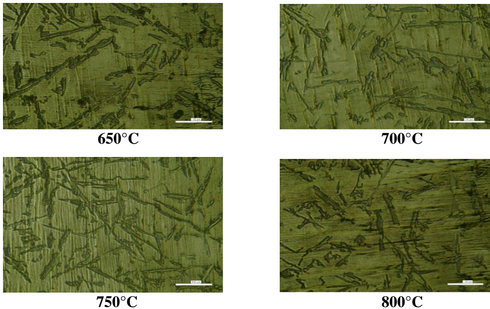
Gambar 18. Hasil Pengujian Mikrostruktur Baling – Baling Kapal Surabaya
