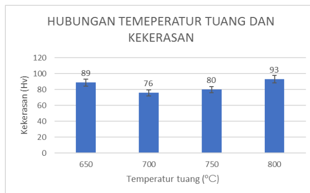
Gambar 14. Hasil Pengujian Kekerasan Baling – Baling Kapal Negara
