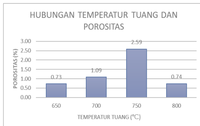
Gambar 16. Hasil Pengujian Porositas Baling – Baling Kapal Surabaya
